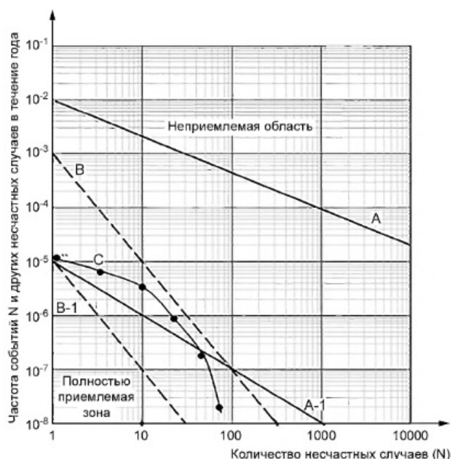
Рисунок Б.15 — Пример диаграммы F-N
