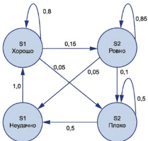
Рисунок Б.7 — Пример диаграммы Маркова
