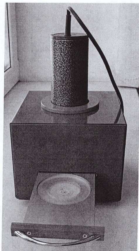
Рисунок 1 - Блок детектирования и устройство для экспонирования
