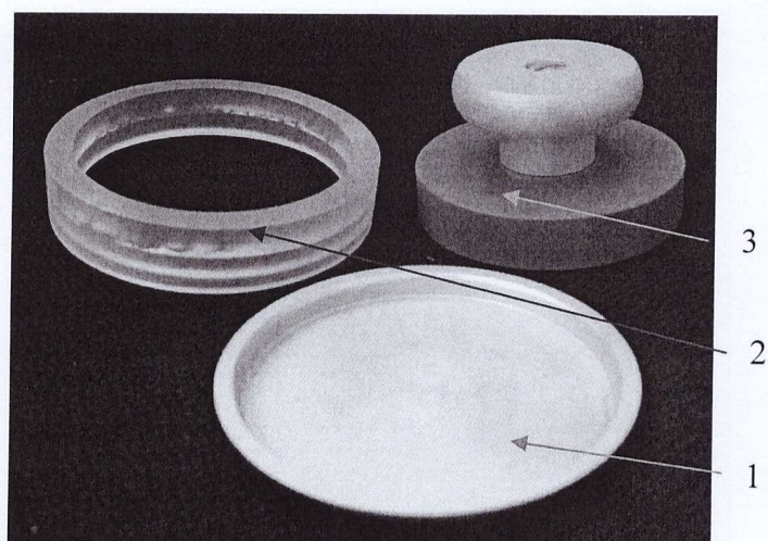
1 – измерительная кювета; 2 – направляющее кольцо 3 – ручной пресс
